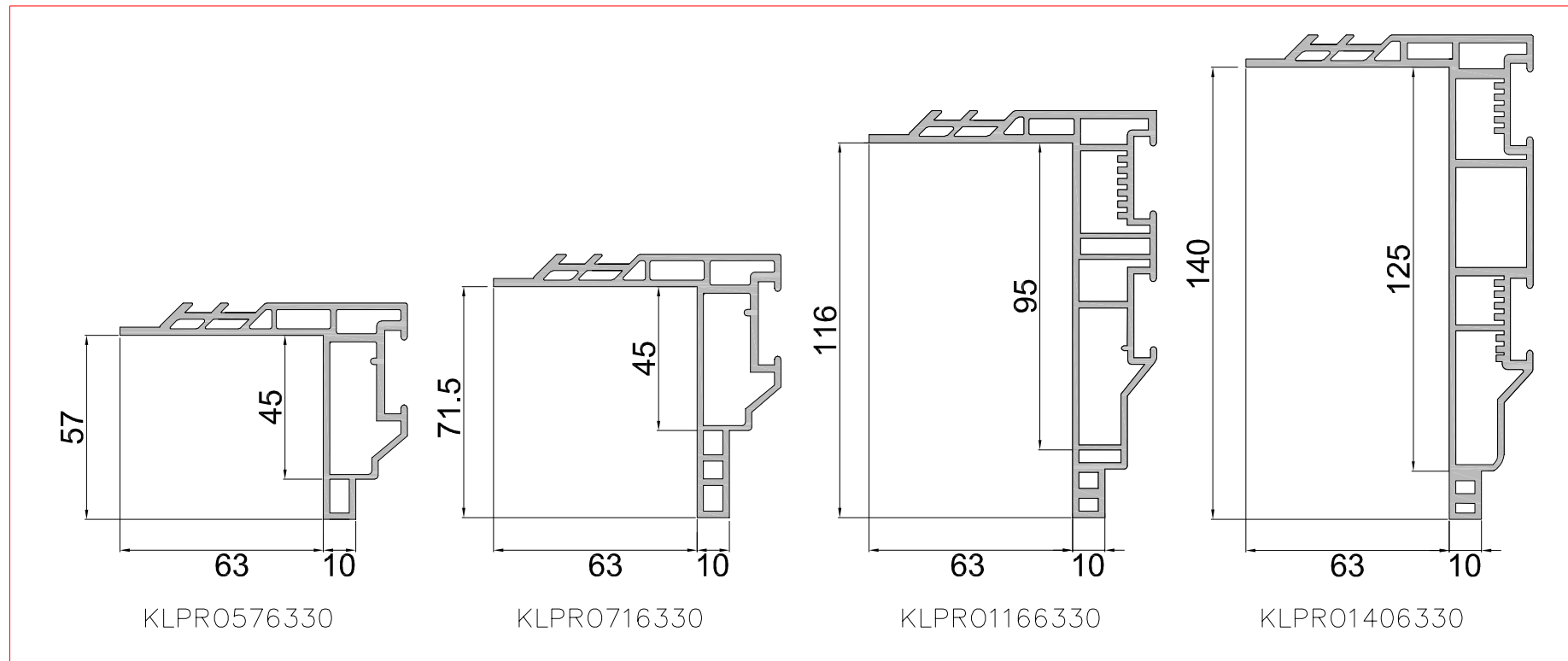
KLIMA PRO CON BATTUTA DA 63
