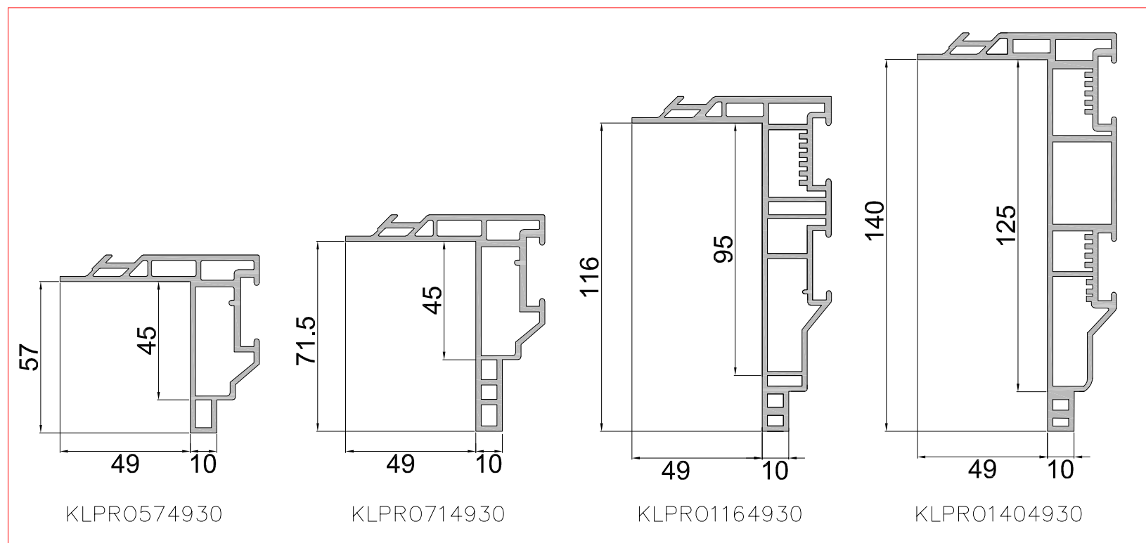
KLIMA PRO CON BATTUTA DA 49
