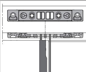
Porta a 2 ante con 2 catenacci
